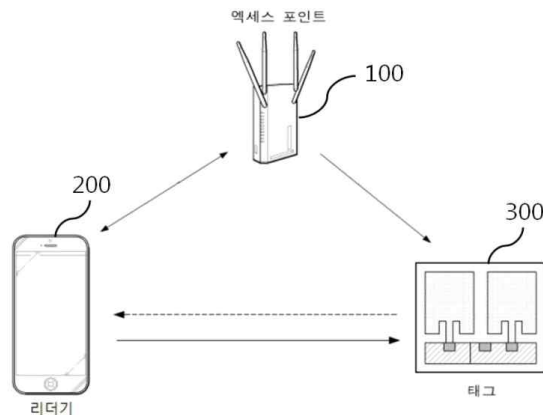
<Wi-Fi 백스캐터 시스템 구성 도면>
